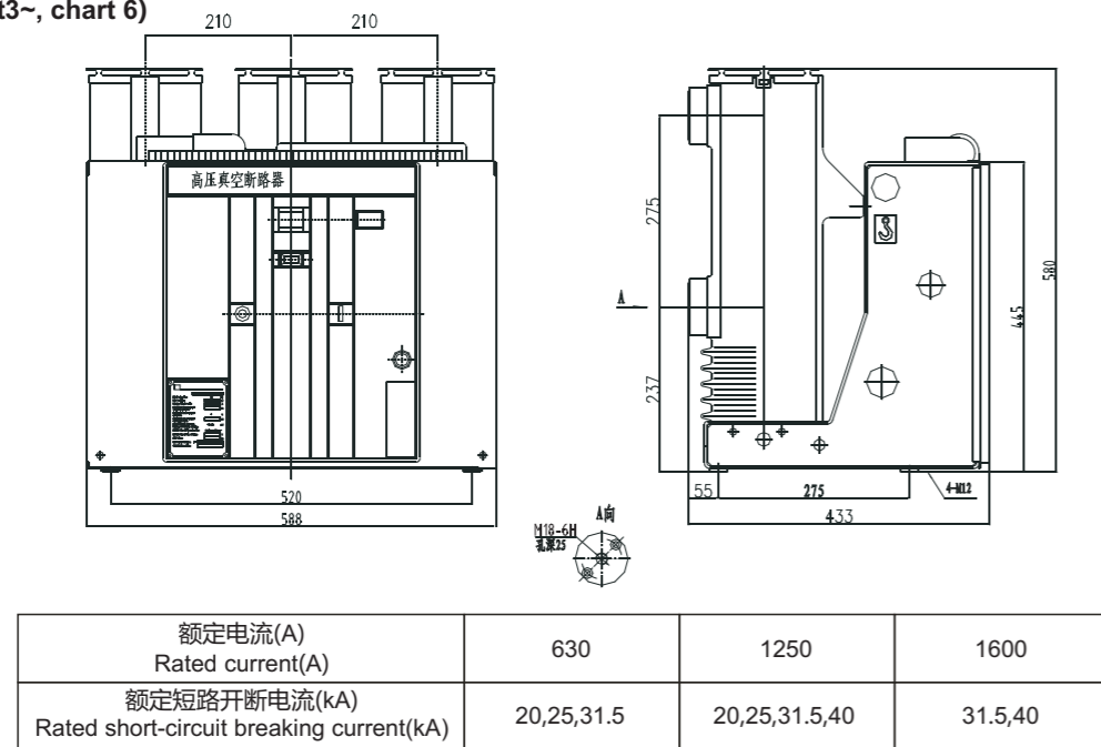
图3 800mm柜固定式断路器外形尺寸 ( 800mm Fixed circait breaker )
